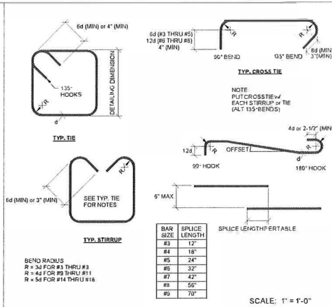
TYP BENDS AND HOOKS 402
